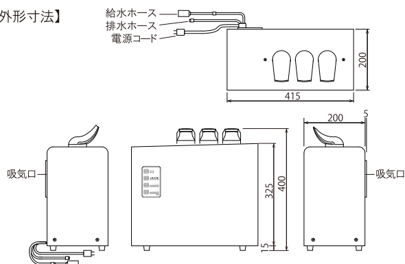
【外形寸法】
